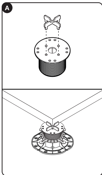
SCREW ŚRUBA
