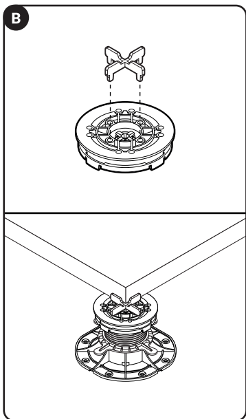
SELF LEVELING HEAD GŁOWICA SAMOPOZIOMUJĄCA
