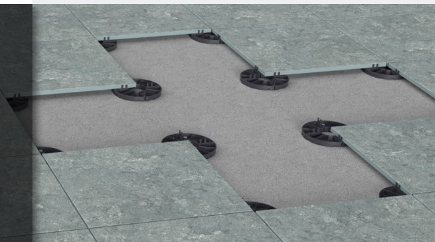
Otworki na motylki dystansowe w podstawkach 8, 10, 15, 16 mm
